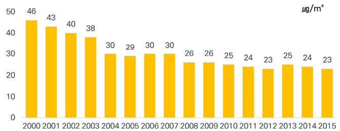
[연도별 초미세먼지(PM-2.5) 농도]
