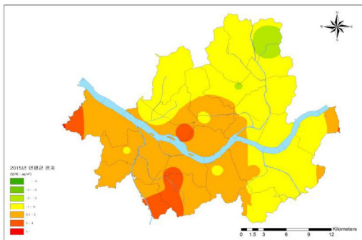
[서울시 지역 PM-2.5 연평균 농도편차 분포(2015년)]
